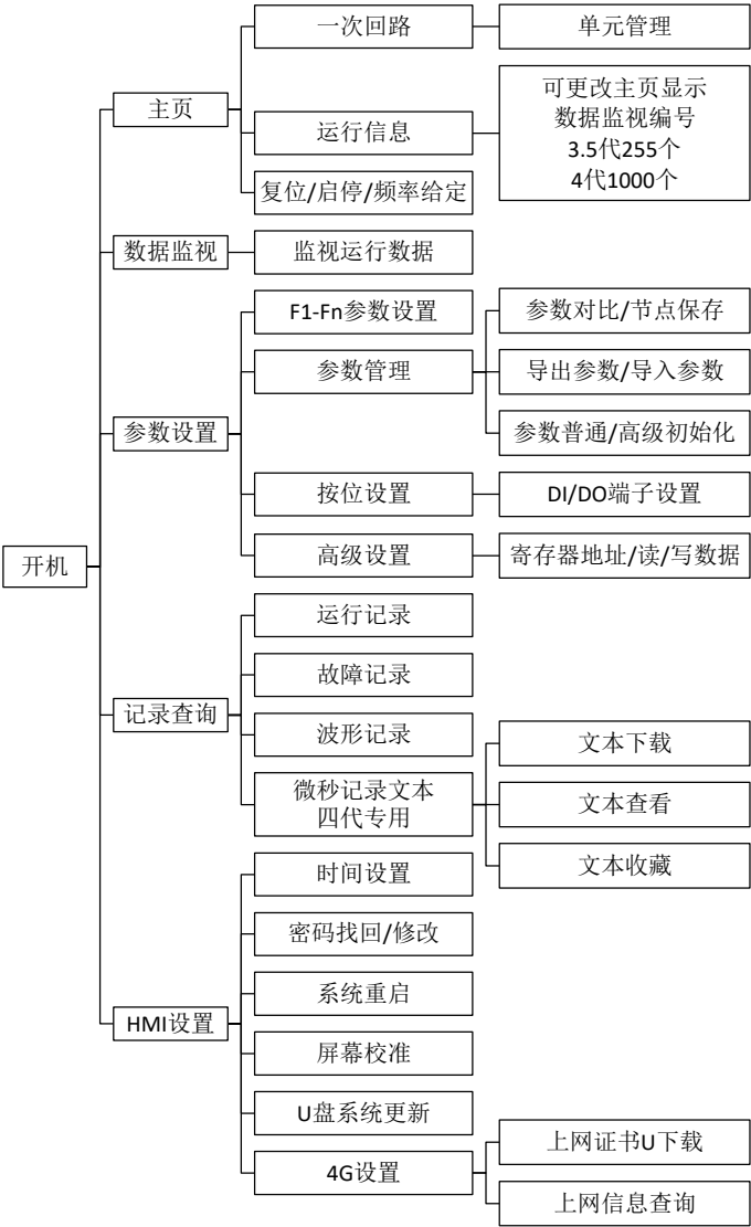
森兰变频高压变频软起原理框图:
